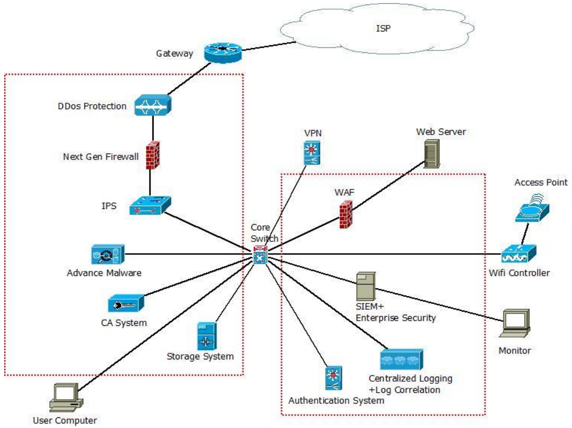
รูปที่ ๑ แนวความคิดการติดตั้งอุปกรณ์และระบบประจำ CSOC ระดับ ๑
