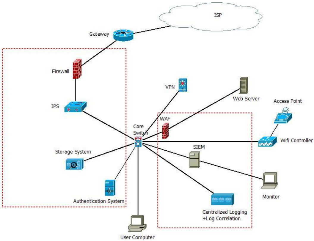
รูปที่ ๒ แนวความคิดการติดตั้งอุปกรณ์และระบบประจำ CSOC ระดับ ๒
