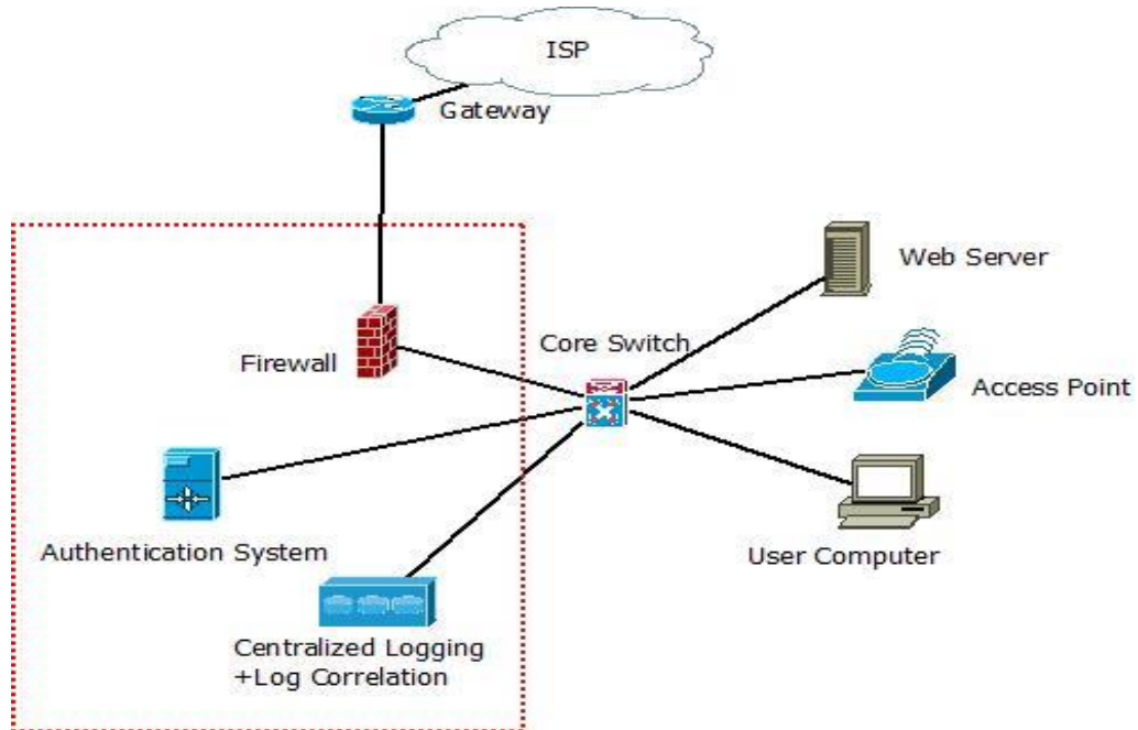
รูปที่ ๔ แนวความคิดการติดตั้งอุปกรณ์และระบบประจำ CSOC ระดับ ๔
