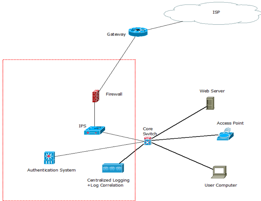
รูปที่ ๓ แนวความคิดการติดตั้งอุปกรณ์และระบบประจำ CSOC ระดับ ๓
